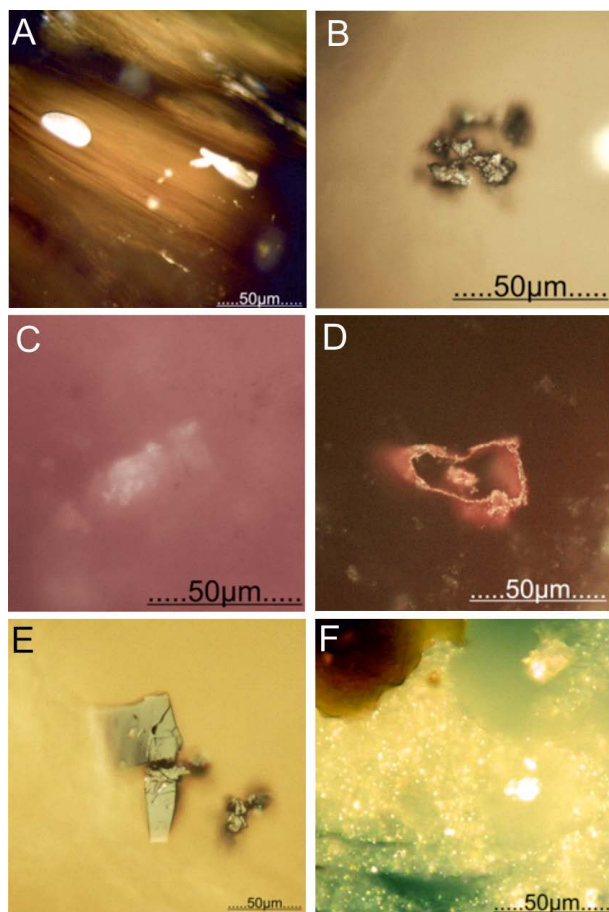
Rys. 5. Identyfikacja zanieczyszczeń w próbce 18.222 pelletu drzewnego w świetle odbitym A – biomasa (pellet drzewny). Zanieczyszczenia: B – metal, C – tworzywo sztuczne, D – rdza, E – węgiel, F – materia mineralna Fig. 5. The contamination identification for 18.222 wood pellet sample, reflected light
