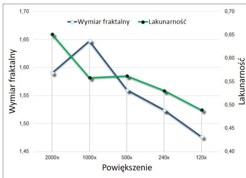
Rys. 7. Zmiana parametrów fraktalnych z rosnącą krotnością powiększenia obrazu dla zdjęcia pojedynczego pora
