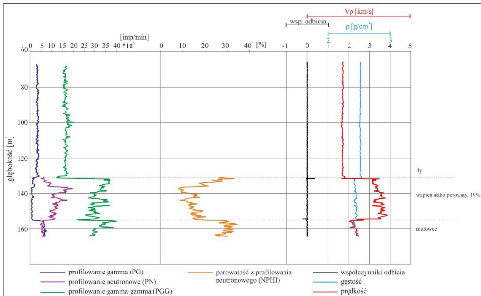
Rys. 3. Zestawienie krzywych geofizyki otworowej dla otworu XX
