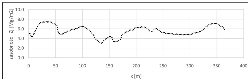
Rys. 8. Rozkład zasobności jednostkowej wzdłuż profilu doświadczalnego (rys. 2)
