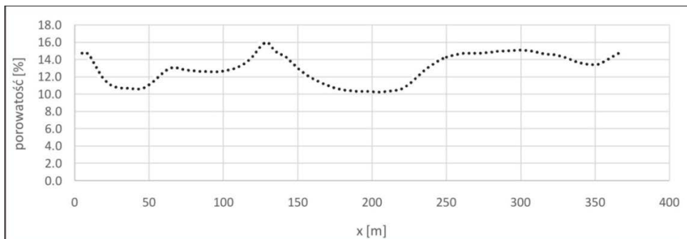
Rys. 6. Rozkład porowatości wzdłuż profilu doświadczalnego (rys. 2)
