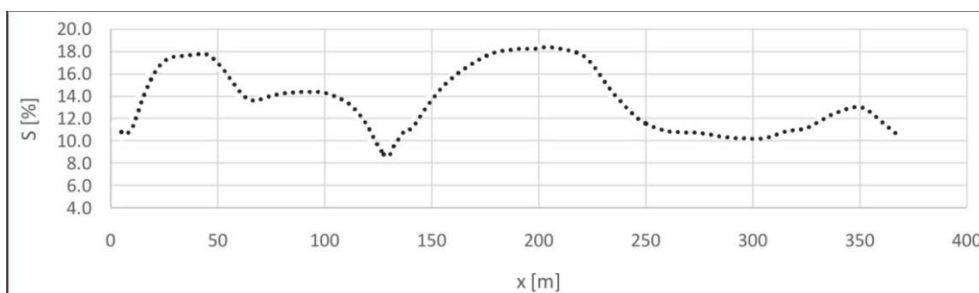
Rys. 7. Rozkład zawartości siarki wzdłuż profilu doświadczalnego (rys. 2)
