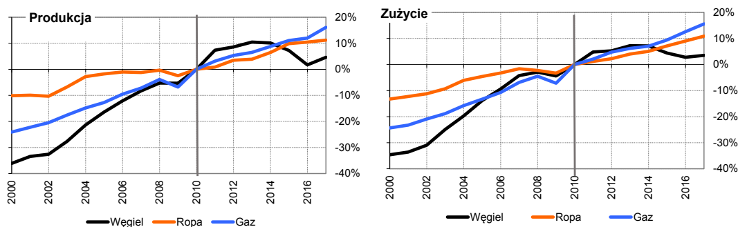
Rys. 3. Porównanie tendencji zmian w produkcji i zużycia głównych nośników energii w świecie Źródło: opracowanie własne na podstawie BP 2018
