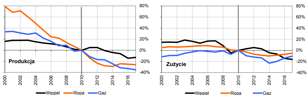
Rys. 4. Porównanie tendencji zmian w produkcji i zużycia głównych nośników energii w UE Źródło: opracowanie własne na podstawie BP 2018
