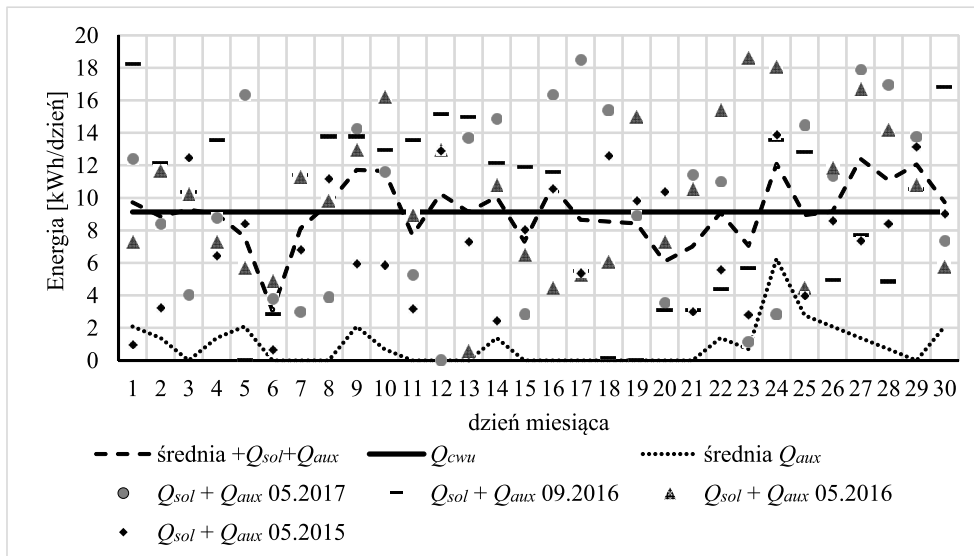
Rys. 2. Wyniki pomiarów ilości ciepła dostarczonego do zasobnika c.w.u. Źródło: opracowanie własne
