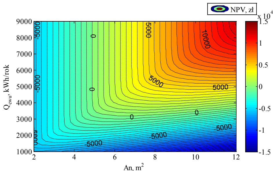
Rys. 6. Suma zdyskontowanych przepływów pieniężnych (NPV) w funkcji powierzchni absorbera oraz zapotrzebowania na ciepło na potrzeby przygotowania ciepłej wody użytkowej ( Q_{cwu} ) Źródło: opracowanie własne
