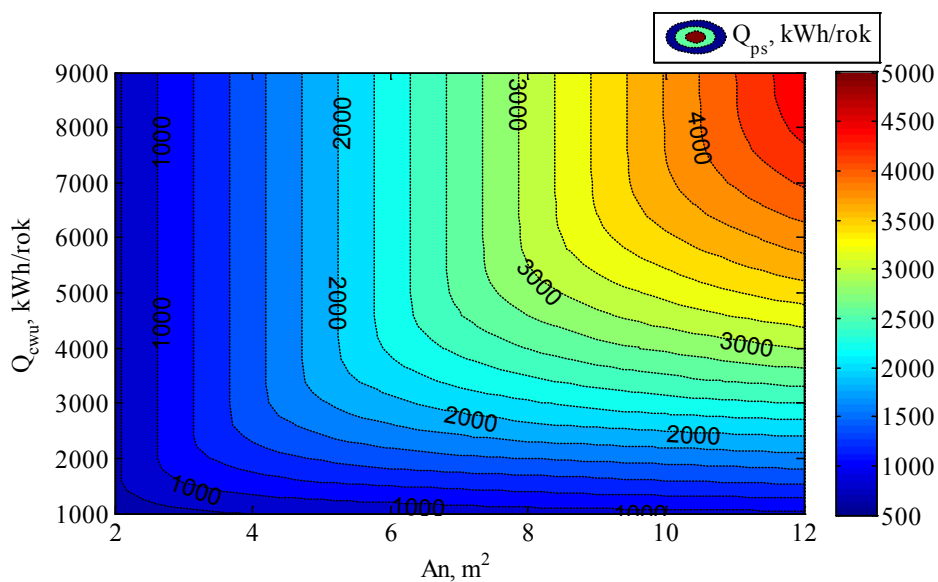
Rys. 5. Efektywne uzyski solarne ( Q_{ps} ) w funkcji powierzchni absorbera ( A_n ) oraz zapotrzebowania na ciepło na potrzeby przygotowania ciepłej wody użytkowej ( Q_{cwi} ) Źródło: opracowanie własne
