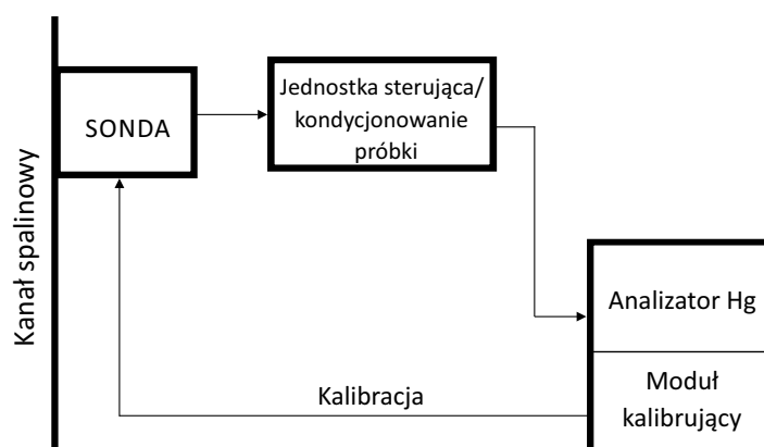
Rys. 1. Schemat Hg-CEMS (na podstawie Zhao i in. 2019)
