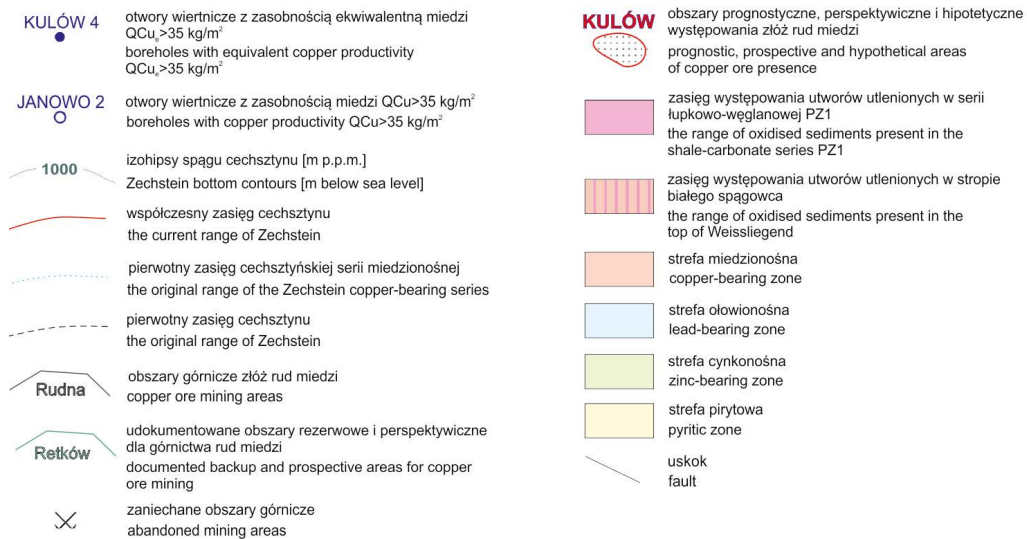
Rys. 1. Obszary o zasobach prognostycznych, perspektywicznych i hipotetycznych występowania rud miedzi przedstawione w Bilansie perspektywicznych zasobów kopalni Polski według stanu na 31 XII 2009 r. (Oszczepalski i Speczik 2011)
