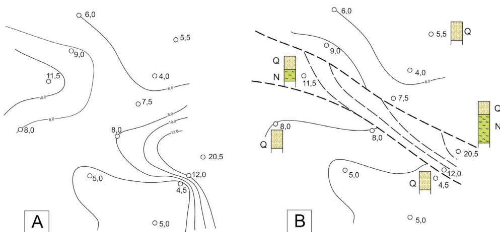
Rys.6. Interpretacja morfologii stropu złoża A – bez uwzględnienia budowy nadkładu, B – z uwzględnieniem budowy nadkadu; Q – utwory czwartorzędowe, N – utwory neogenu (Nieć 2016)
