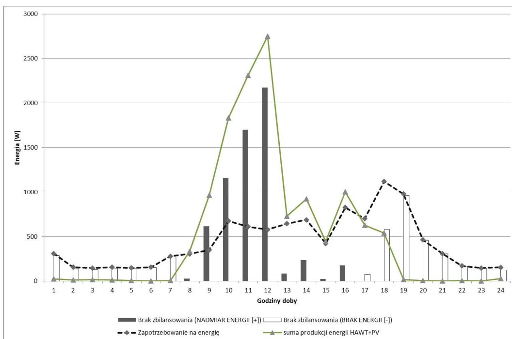
Rys. 4. Bilans zużycia i produkcji energii – dzień 1
