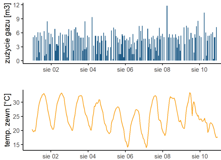
Rys. 3. Godzinowe zużycie gazu w kotłowni A5 w okresie 1–9 sierpnia 2018 r.
